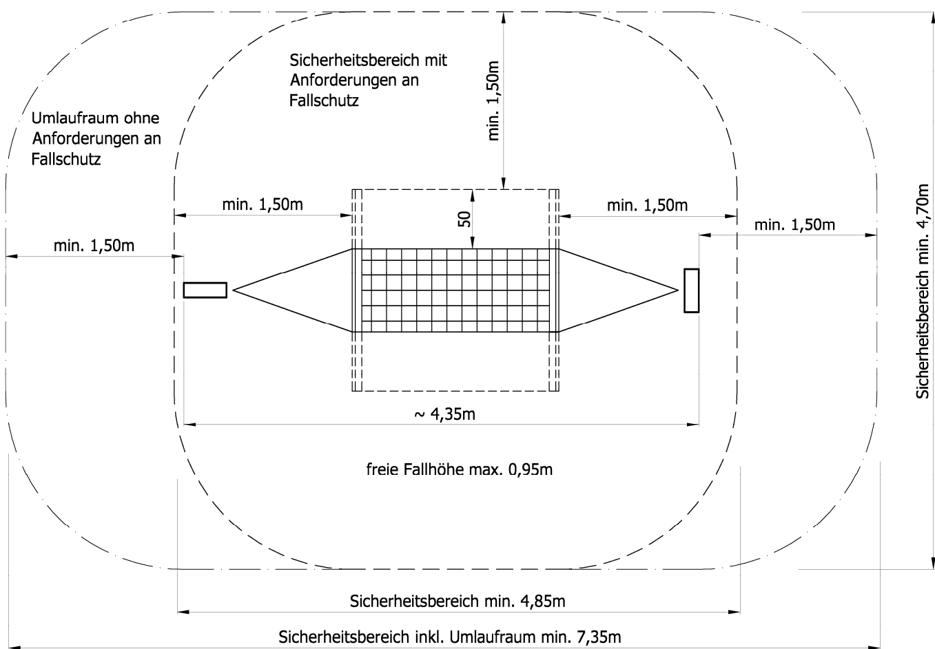
DRAUFSICHT
